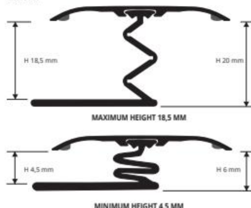
PMPFX... 42090AS / 42A + PMFIXBSAN 23 scale 1:1
