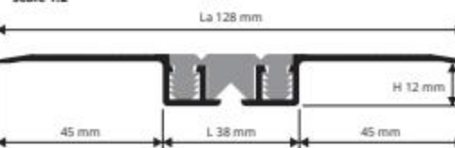
PENF 130... scale 1:2
