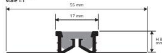
PFXAL/OT 08 scale 1:1
