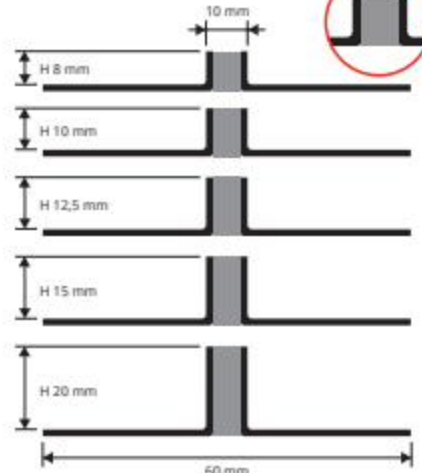
GCAC 125... scale 1:2
