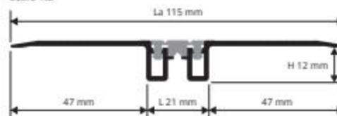
PENF 130... scale 1:2
