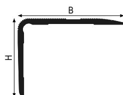
Aluminum SE 45
