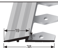
330 EB \varnothing 3 mm offen gestanzt open punched estampé ouvert
