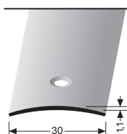
453 mittig versenkt gebohrt centrally countersunk drilled à percement noyé central
