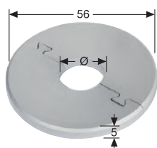
739 ♦ Aluminium Heizrohrrosette aluminium heating tube rosette Rosaces pour tuyaux de chauffage
