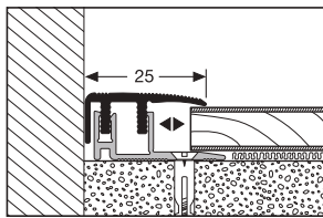
587 XL H \updownarrow 8 - 12 mm
