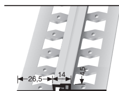
318 G \updownarrow 4,5 mm geschlossen gestanzt punched base estampé fermé
