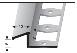
RC100 G \updownarrow 6 - 10 mm geschlossen gestanzt punched base estampé fermé
