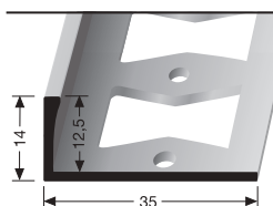
335 G ⇅ 12,5 mm geschlossen gestanzt punched base estampé fermé
