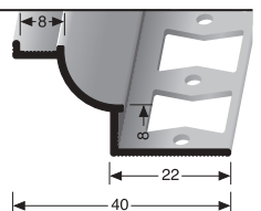
CC080 G 8 mm geschlossen gestanz punched base estampé fermé
