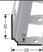
160 G geschlossen gestanz punched base estampé fermé
