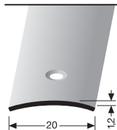
450 ♦ mittig versenkt gebohrt centrally countersunk drilled à perçement noyé central
