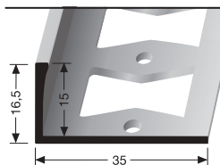
336 G ⇅ 15 mm geschlossen gestanzt punched base estampé fermé
