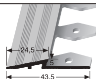
332 EB \varnothing 5 mm offen gestanzt open punched estampé ouvert
