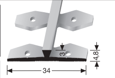
365 EB ± 3 mm offen gestanzt open punched estampé ouvert
