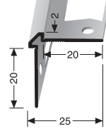
155 G geschlossen gestanz punched base estampé fermé
