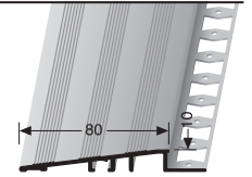
PR100 G \updownarrow 10 mm geschlossen gestanzt punched base estampé fermé
