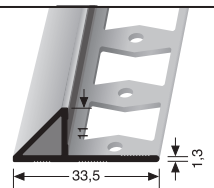
TC110 G 11 mm geschlossen gestanz punched base estampé fermé
