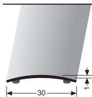
451 SK selbstklebend self-adhesive auto-adhésif
