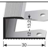
213 EB \varnothing 12 - 13,2 mm offen gestanzt open punched estampé ouvert
