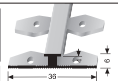
366 EB ± 4 mm offen gestanzt open punched estampé ouvert
