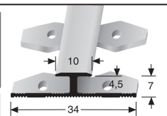
368 EB ± 4,5 mm offen gestanzt open punched estampé ouvert
