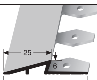
333 EB \varnothing 5,5 - 6 mm offen gestanzt open punched estampé ouvert
