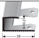
212 EB \varnothing 9 - 10,2 mm offen gestanzt open punched estampé ouvert
