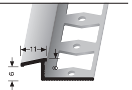
RC080 G \updownarrow 6 - 8 mm geschlossen gestanzt punched base estampé fermé
