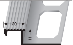
TR110 G \updownarrow 11 mm geschlossen gestanzt punched base estampé fermé
