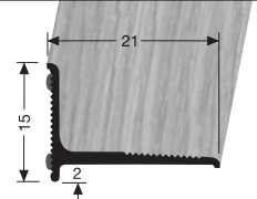
369 H/SK mit Holzdekor, selbstklebend with wood decor, self-adhesive avec décor bois, auto-adhésif
