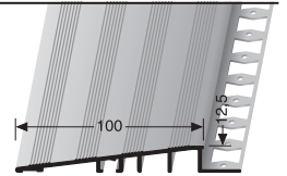
PR125 G \updownarrow 12,5 mm geschlossen gestanzt punched base estampé fermé
