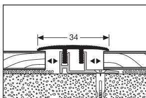
588 XL H \updownarrow 8 - 12 mm
