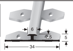
363 EB ± 2,5 mm offen gestanzt open punched estampé ouvert
