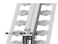
323 G \updownarrow 12,5 mm geschlossen gestanzt punched base estampé fermé
