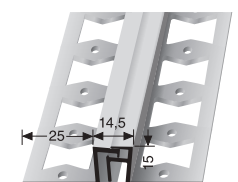
324 G ♦ \updownarrow 15 mm geschlossen gestanzt punched base estampé fermé
