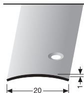
471 S ♦ seitlich versenkt gebohrt laterally countersunk drilled à perçement noyé latéral
