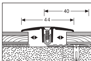
388 XXL \updownarrow 7 - 18 mm*
