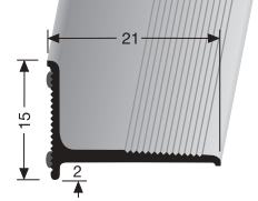
369 SK selbstklebend self-adhesive auto-adhésif
