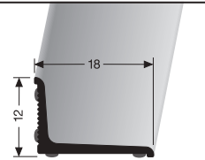
369N/SK selbstklebend self-adhesive auto-adhésif
