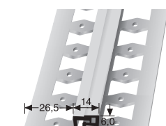
319 G \updownarrow 6 mm geschlossen gestanzt punched base estampé fermé
