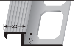
TR090 G \updownarrow 9 mm geschlossen gestanzt punched base estampé fermé
