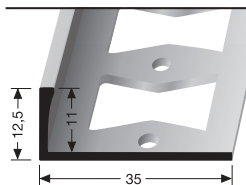
338 G ⇅ 11 mm geschlossen gestanzt punched base estampé fermé
