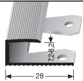
210 EB \varnothing 7,2 - 8,2 mm offen gestanzt open punched estampé ouvert
