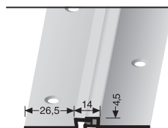
318 SK \updownarrow 4,5 mm selbstklebend self-adhesive auto-adhésif
