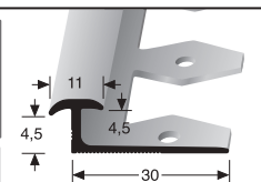
345 EB ± 4,5 mm offen gestanzt open punched estampé ouvert
