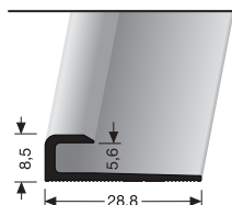
799 U \varnothing 5,6 mm
